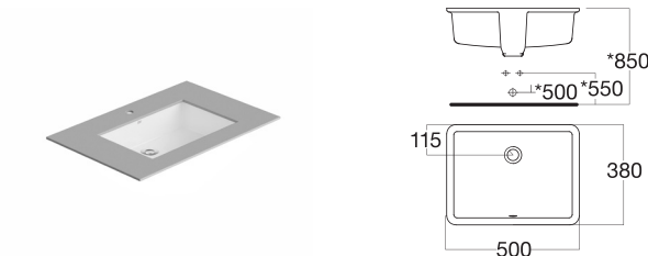
Chậu rửa âm bàn
