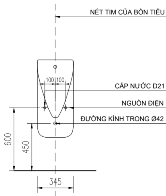
CHI TIẾT CẤP CHỜ BỒN TIỂU TREO BU-14018S
