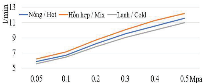
Lưu lượng miệng xả / Aerator's flowrate chart
